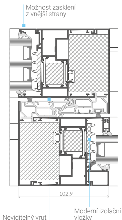
Řez středového sloupku
